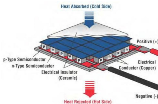
Fig. 4.1 Thermoelectric Module
