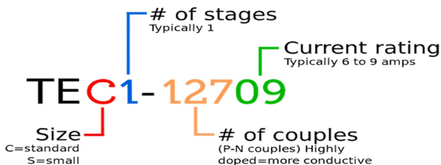
Fig .4.2 TEC
