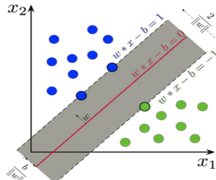
Fig.1.A typical Linear SVM classifier
