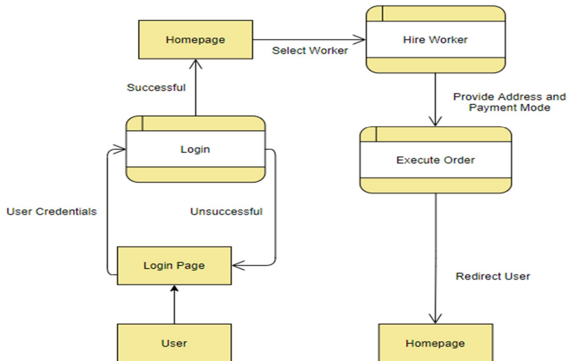
Level 1 DFD
