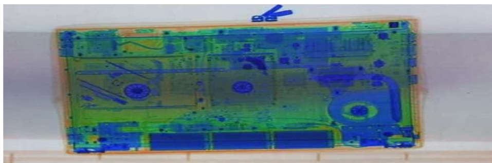
Fig.1 : CLAHE OUTPUT
