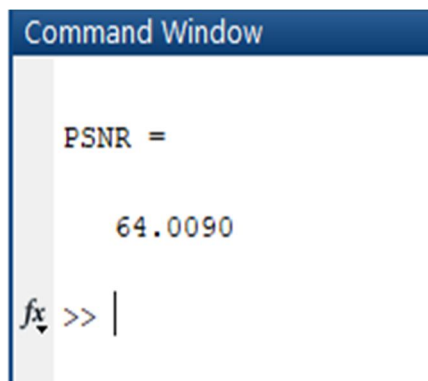
Fig. 5. PSNR
