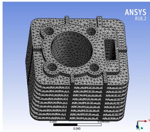
Fig.3 Fins meshing Al 6061 materials meshing
