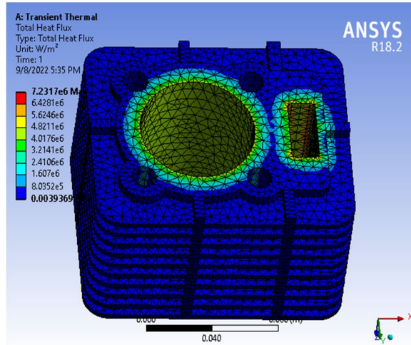
Fig. 12: Fins Al 6061 materials total heat flux at 500°C transient
