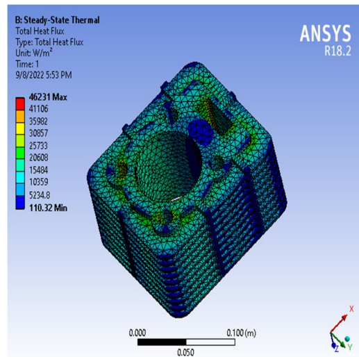
Fig. 7 : Fins Al 6061 materials total heat flux at 300 0 C steady
