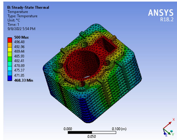
Fig. 15 : Fins Al 6061 materials temperature at 500 0 C steady
