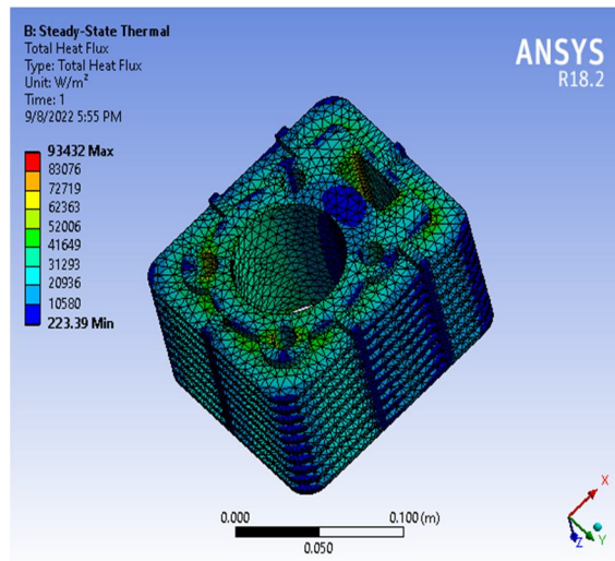
Fig. 13 : Fins Al 6061 materials total heat flux at 500°C steady
