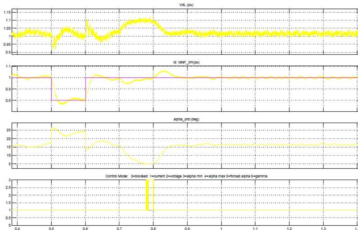
Fig. 4 Rectifier DC quantities
