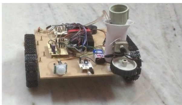
Fig.12 BOT
