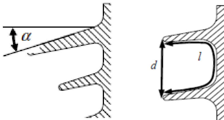
Fig.4 Shed angle ( \alpha ) and spacing (d)
