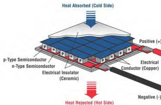
Fig. 4.1 Thermoelectric Module
