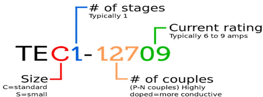
Fig. 4.2 TEC
