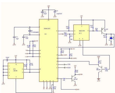
Fig. 8. Microntroller Interface
