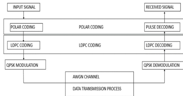
Fig.9. NR Polar Coding System
