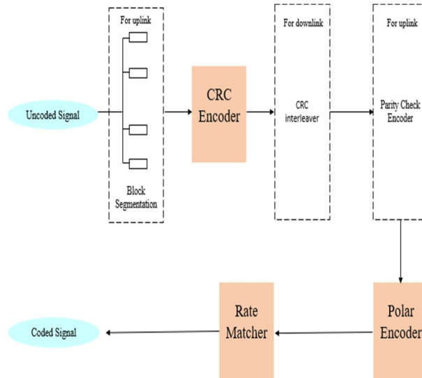
Fig.9. NR Polar Coding System
