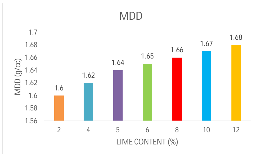
Figure 3. MDD w. r. t. Lime
