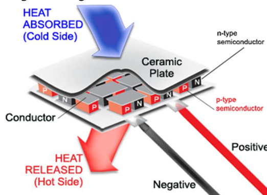
Fig. 2 Thermoelectric module
