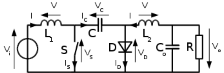
Fig: 4 Cuk Converters
