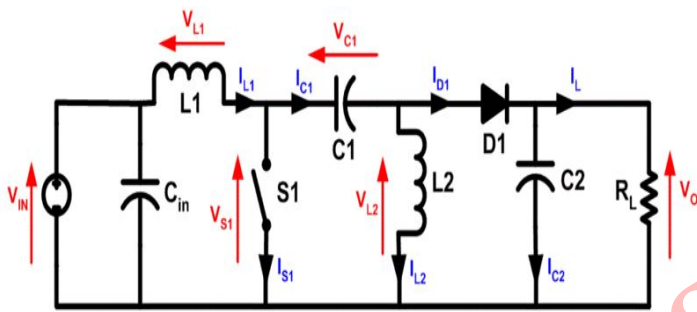
Fig: 5 SEPIC converter
